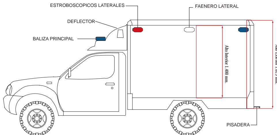
VISTA LATERAL
